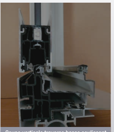
Coupe verticale traverse basse coulissant avec seuil standart RT 2012
